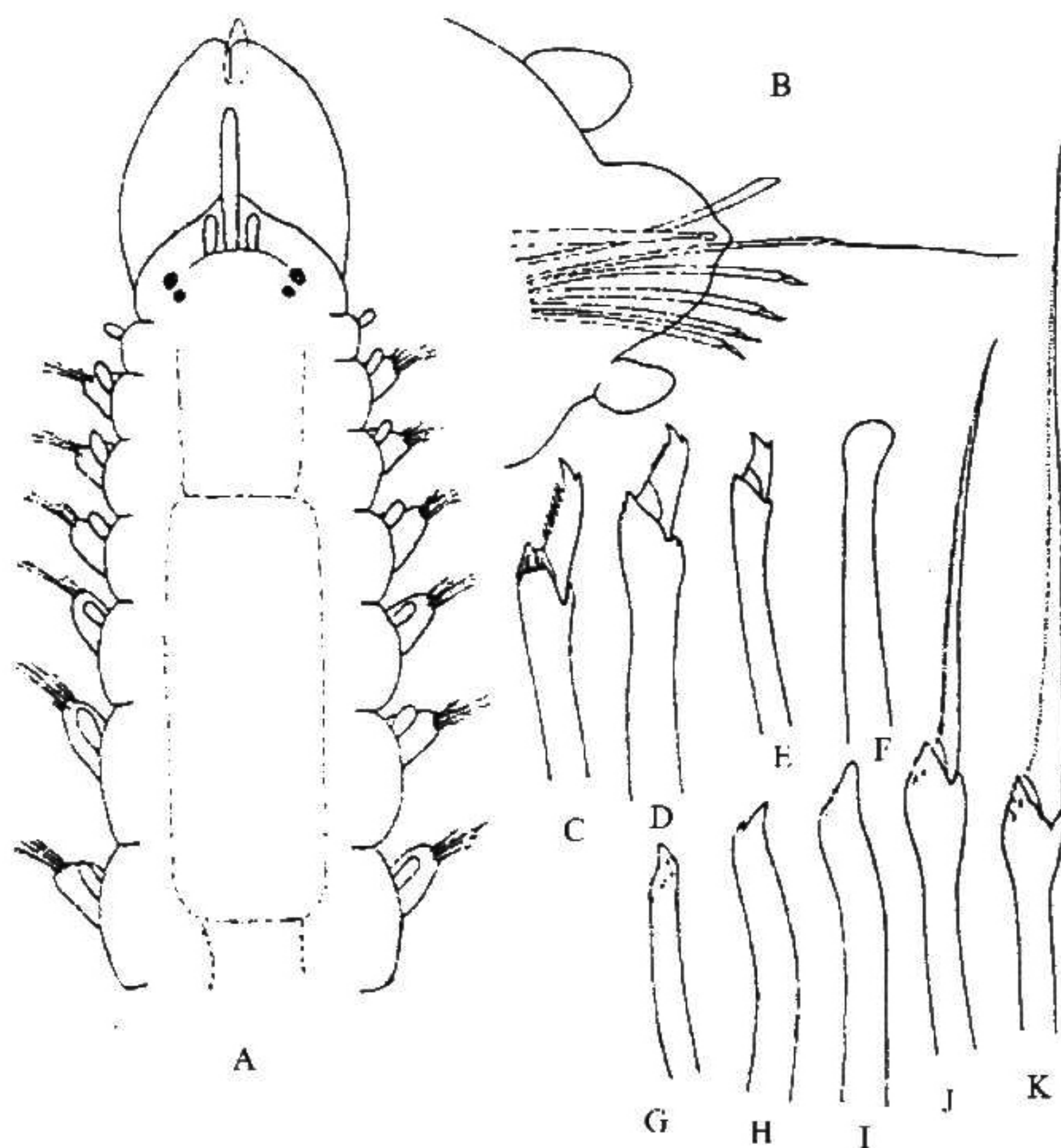
图 154 不等艾裂虫 Exogone dispar (Webster)
